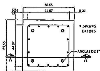
PLANTA - DADO DE CIMENTACIÓN
