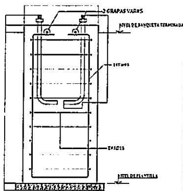
ALZADO - DADO DE CIMENTACIÓN CORTE A-A
